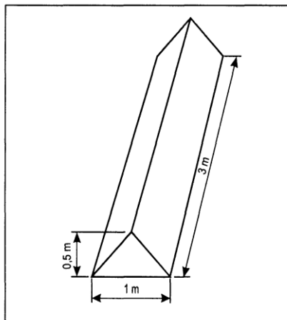
Figura 5 -32. Balizas delimitadoras
